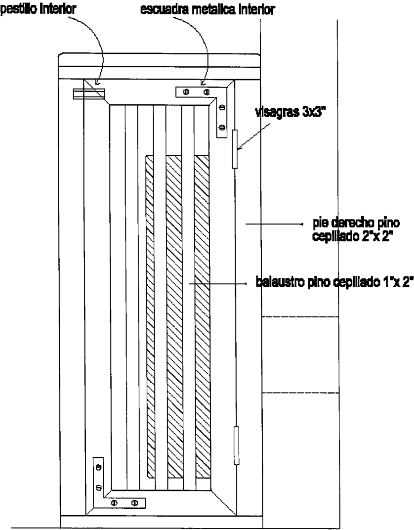
ELEVACION LATERAL
