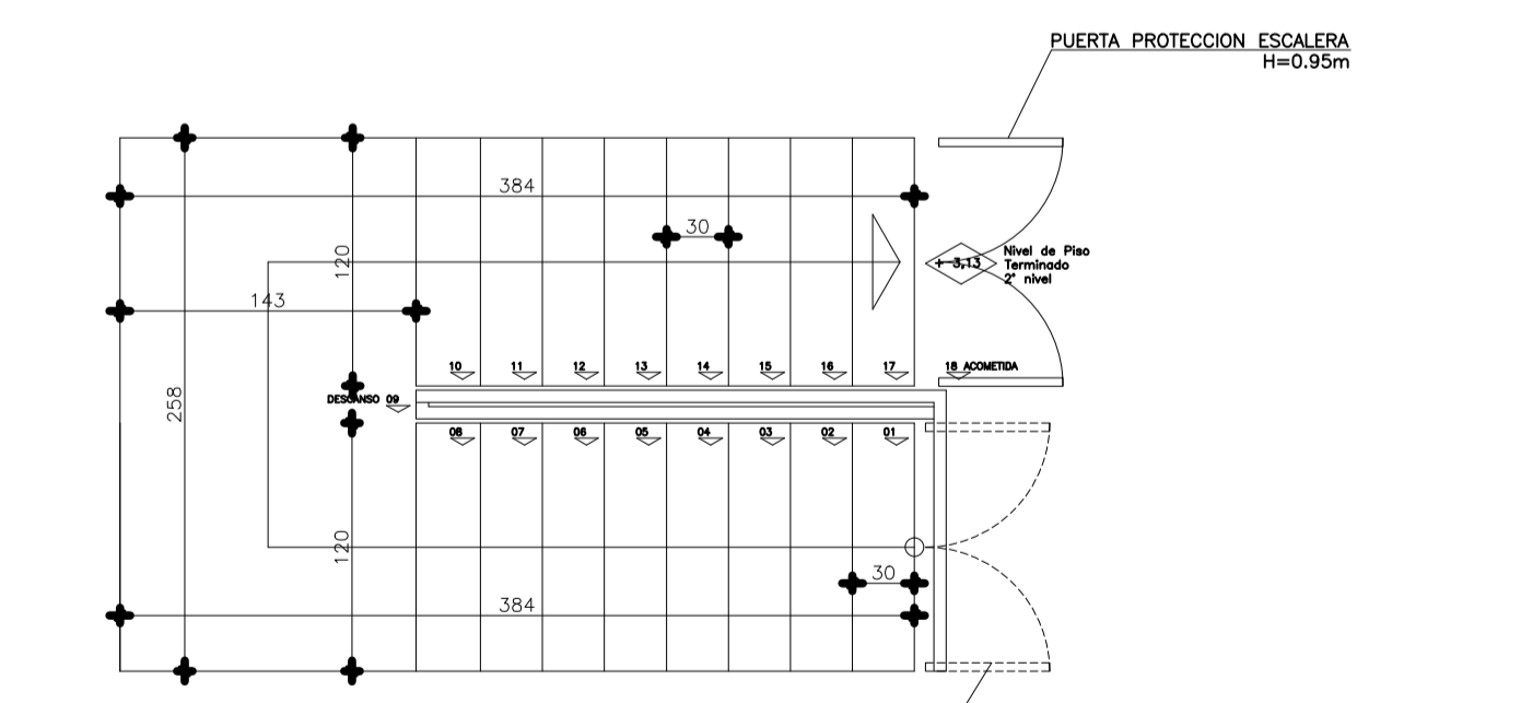
Planta Escalera Interior
