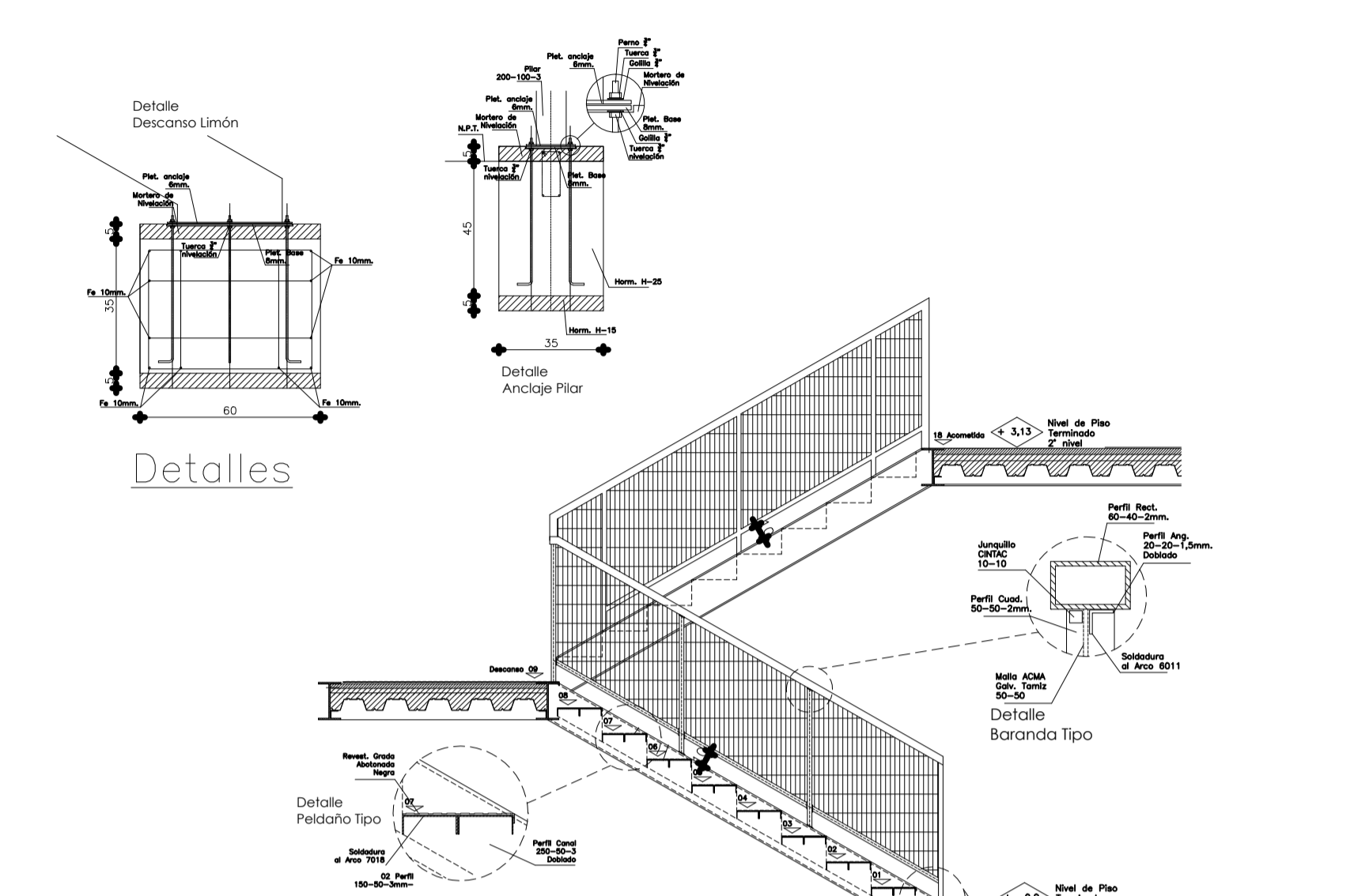
Corte Constructivo
