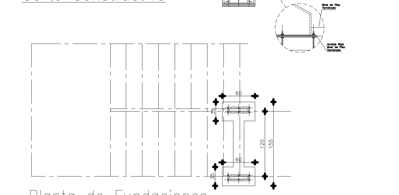
Planta de Fundaciones
