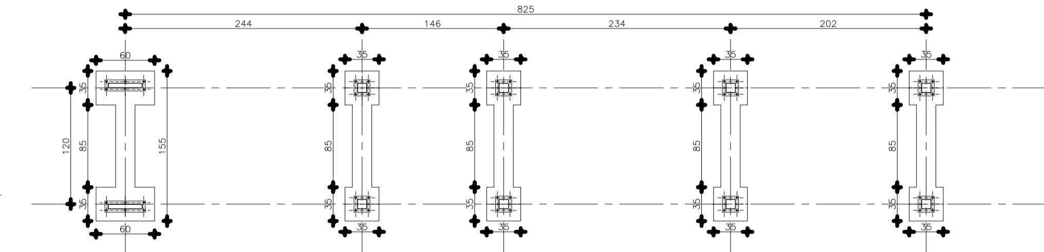
Planta de Fundaciones
