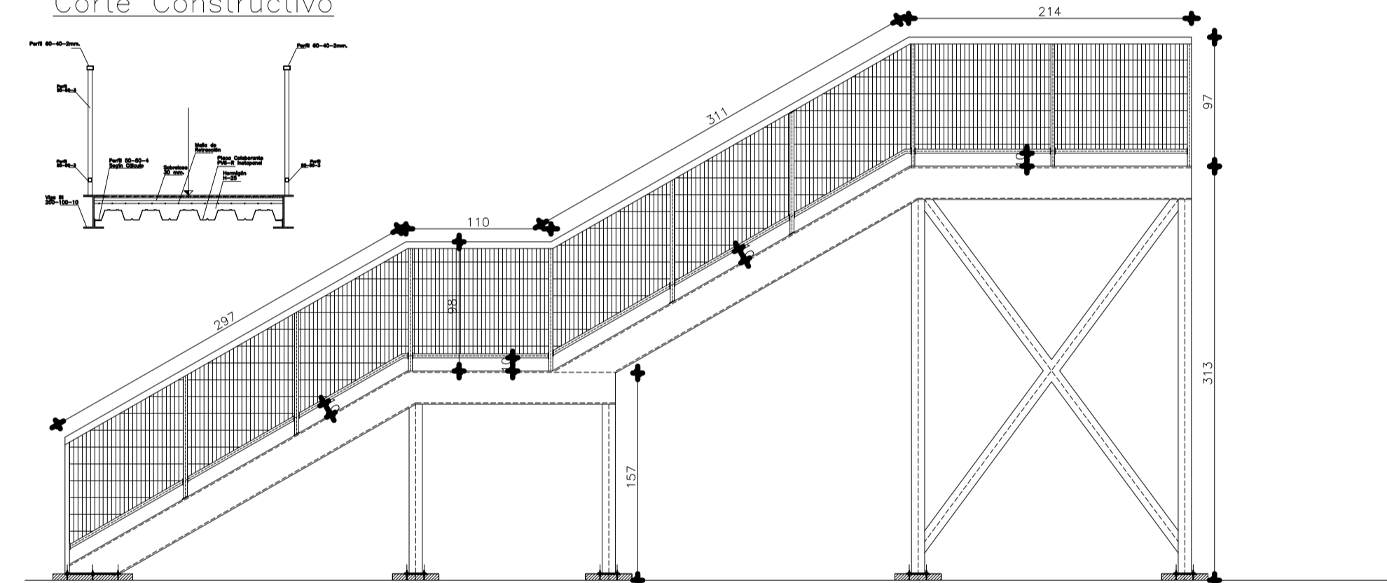
Elevación
