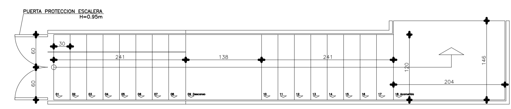
Planta Escalera Exterior
