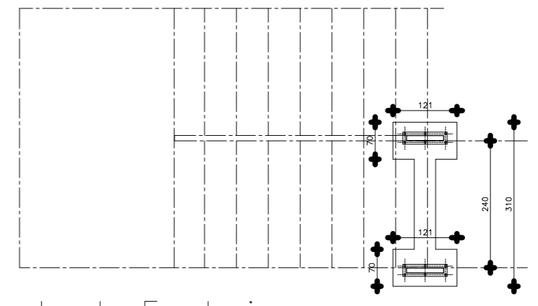
Planta de Fundaciones
