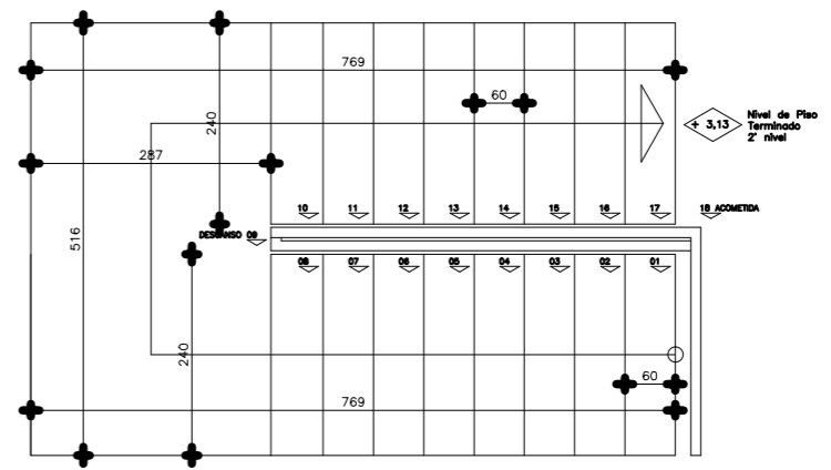
Planta Escalera Interior
