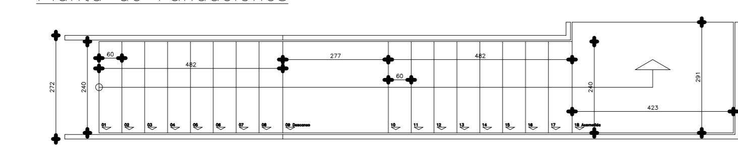
Planta Escalera Exterior
