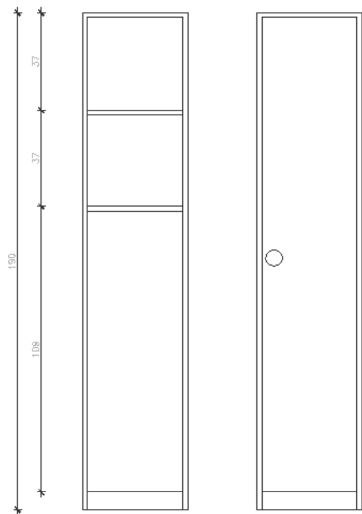
mueble aseo
