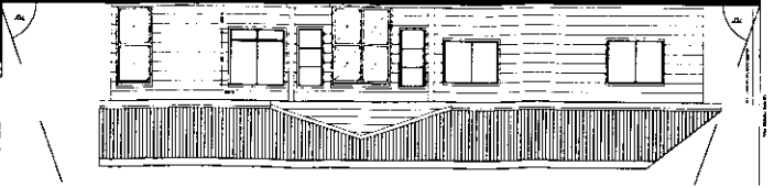
ELEVACION SUR ESC. 1:50
