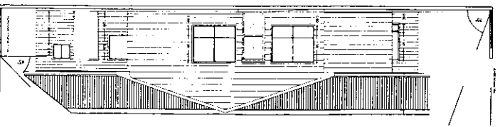
ELEVACION SUR ESC. 1:50
