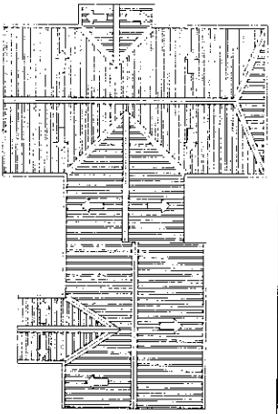
PLANTA DE CUBIERTA ESC. 1:100
