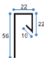
Perfil J universal
