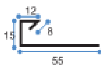
Perfil alero
