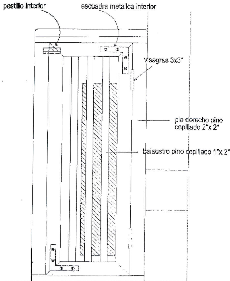
ELEVACION LATERAL
