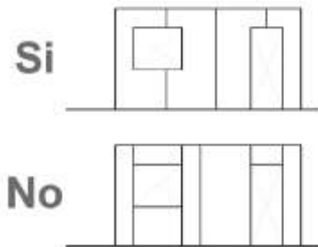
Esquema instalación de placas sobre vanos:
