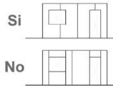
Esquema instalación de placas sobre vanos:
