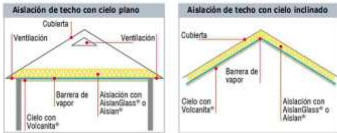
REGLEMENTACIÓN TÉRMICA OBLIGATORIA PARA TECHUMBRE, MUROS Y PISOS VENTILADOS (SEGUN ORDENANZA GENERAL DE URBANISMO Y CONSTRUCCIONES).
