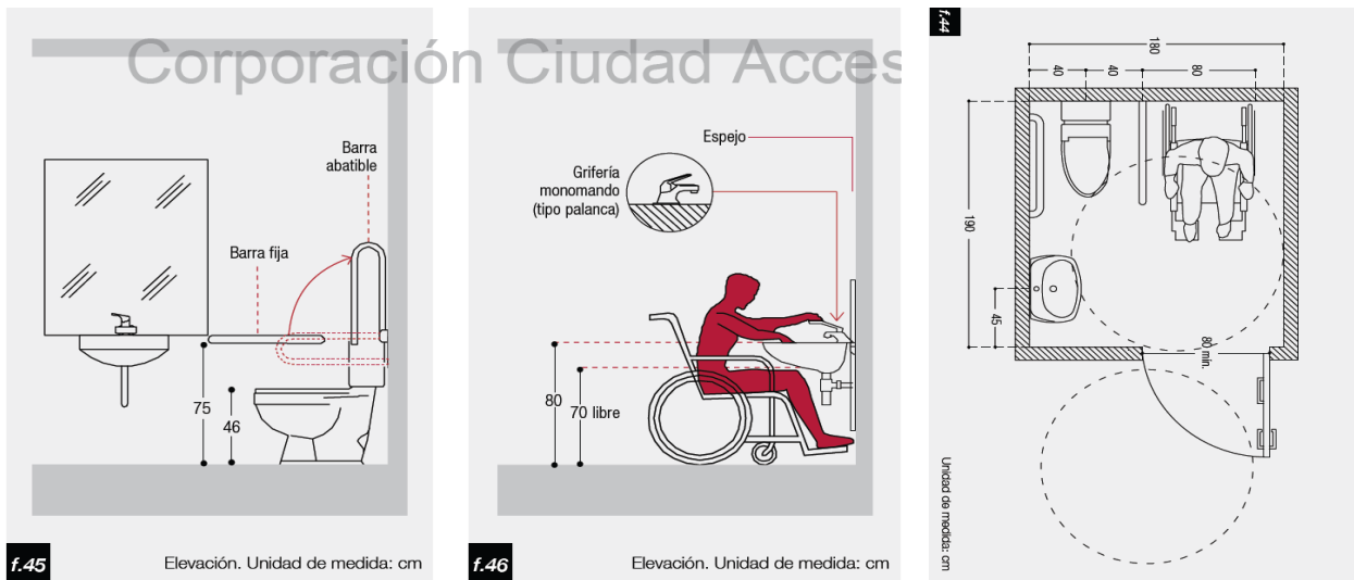
f.45 Elevación. Unidad de medida: cm
