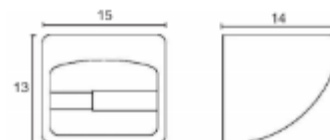
PORTARROLLO WEIS CH6030001 • Aluminio • Porcelana vitrificada
